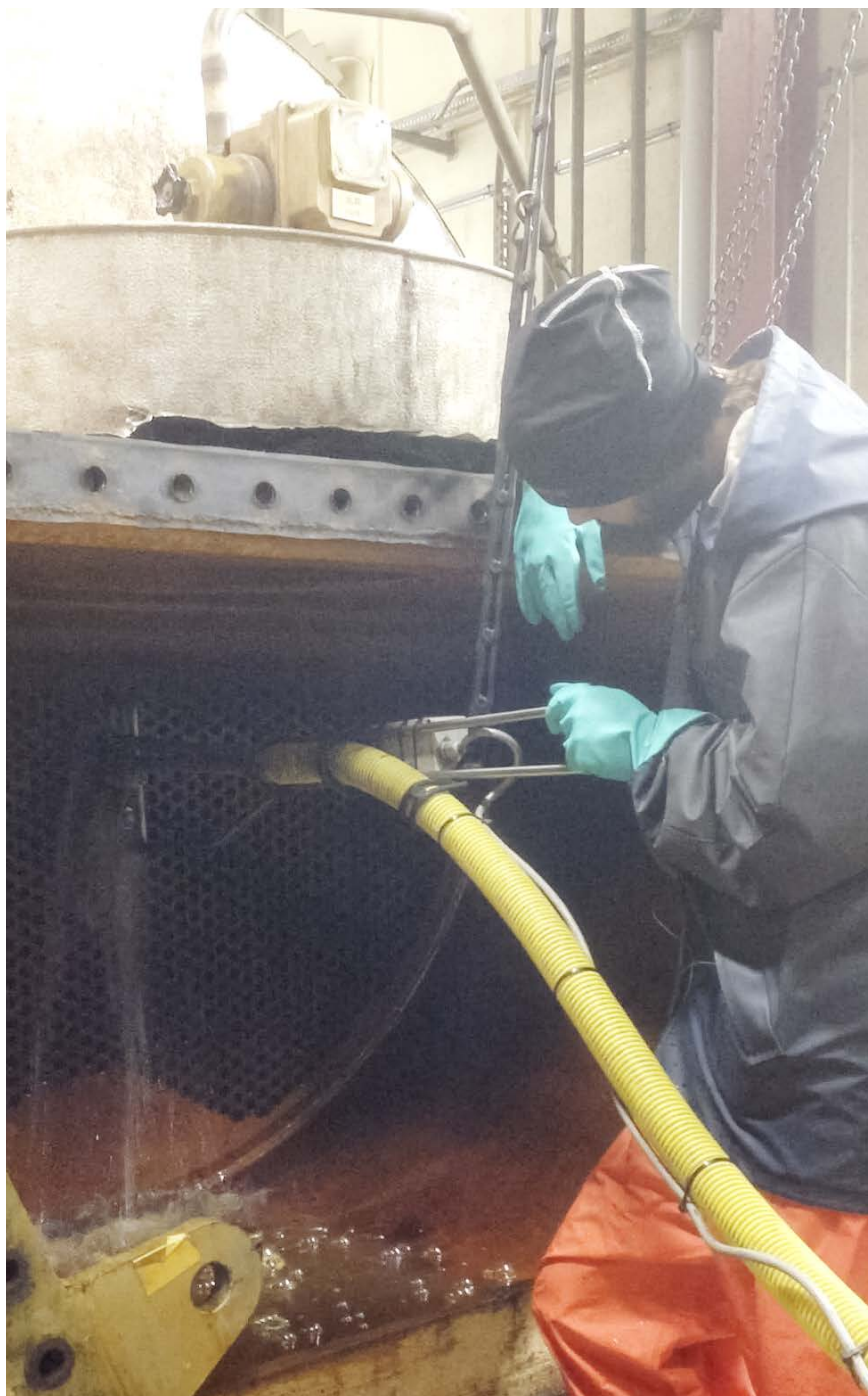
Tvätt av stora värmeväxlare i samarbete med Vattenfall. Operatören fäster munstycket från roboten i hålen som ska tvättas. Därefter sker tvätt med iller som matas ut automatiskt i jämn hastighet. Operatören slipper bli nersmutsad av tvättvatten och tvättresultatet blir jämnare och bättre.
